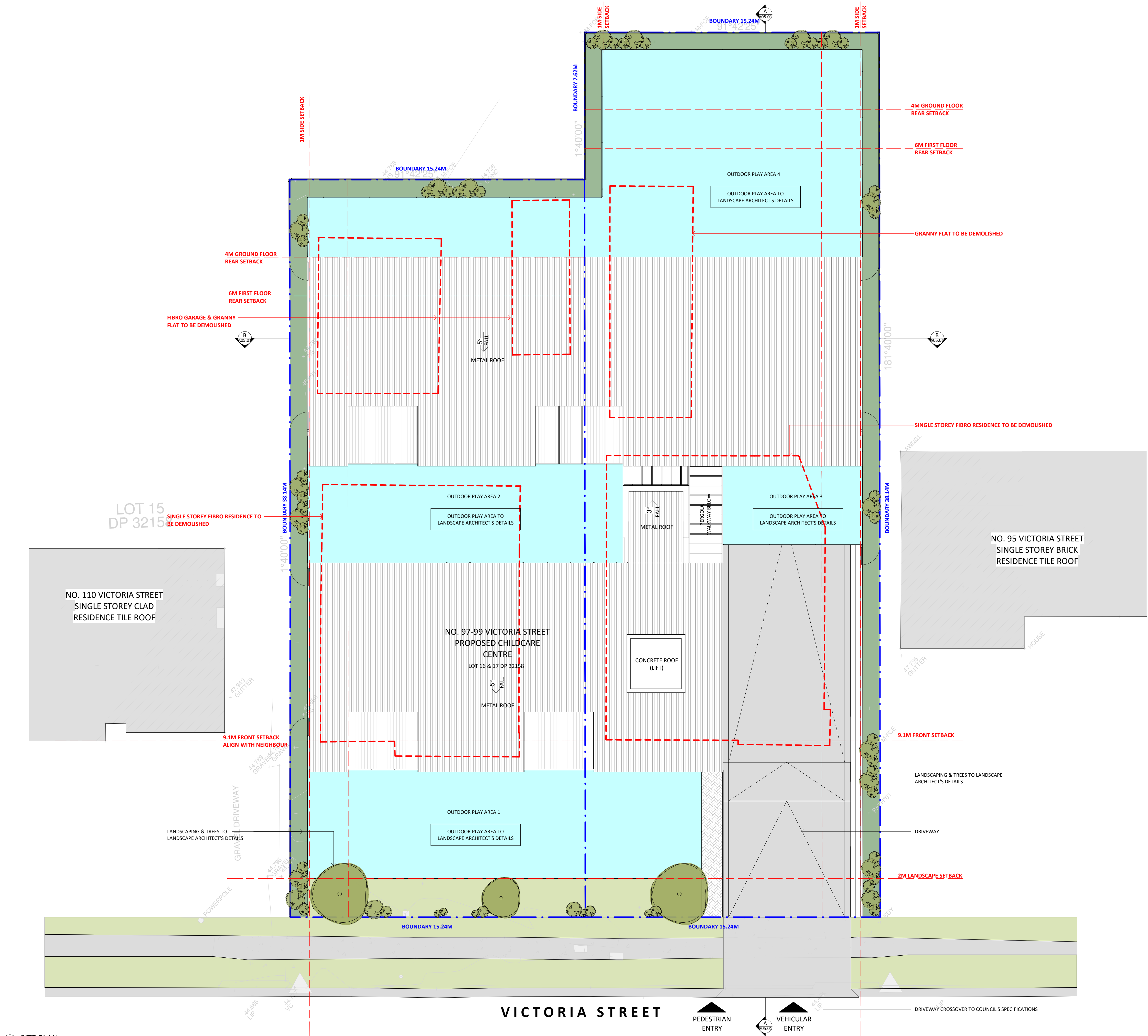
1 SITE PLAN 1:100
