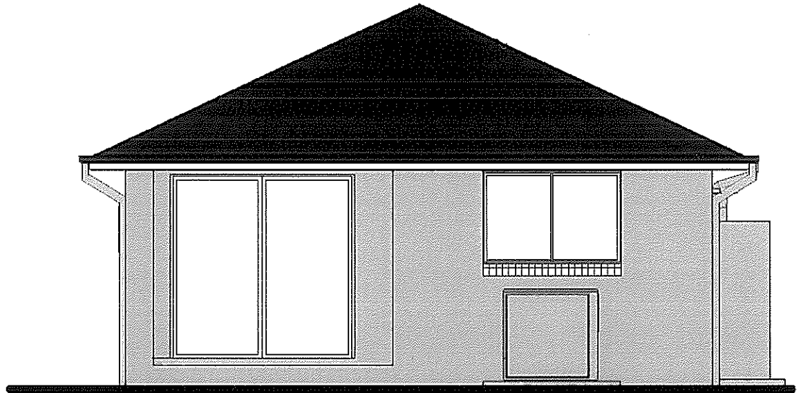
ELEVATION B
