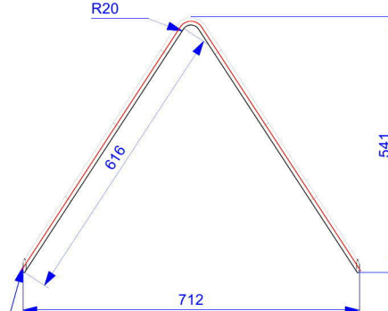
1051/4 Brace Rod
