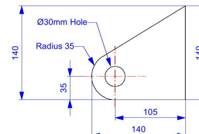
1051/3 Wire Lug
