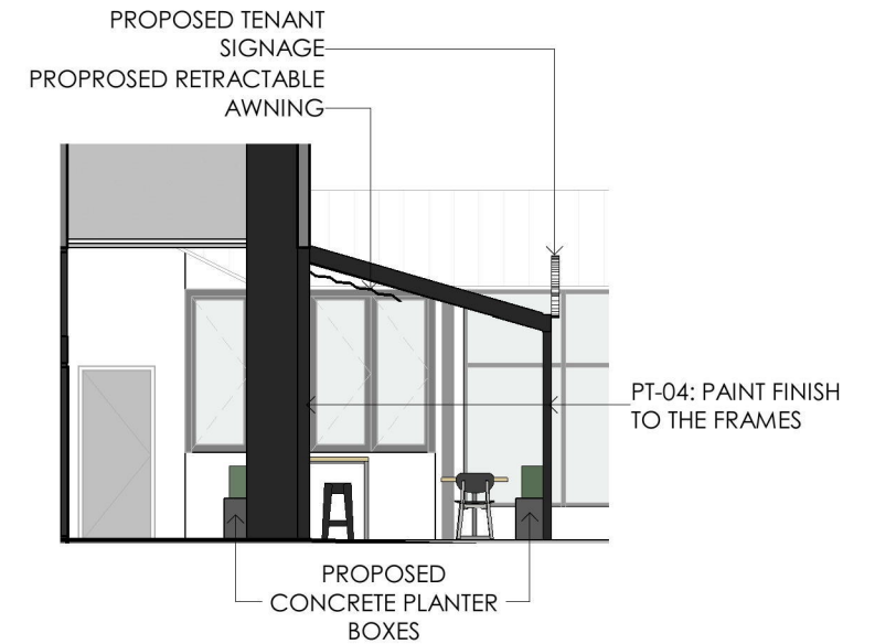
3 ELEVATION 3 DA-03 Scale: 1 : 100
