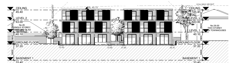
5 NP - NORTH ELEVATION N.T.S
