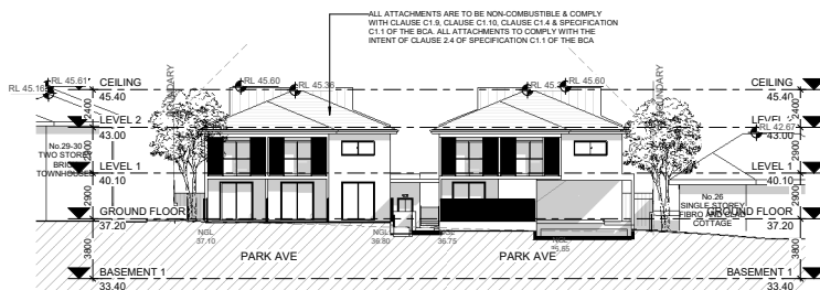
4 NP - SOUTH ELEVATION N.T.S
