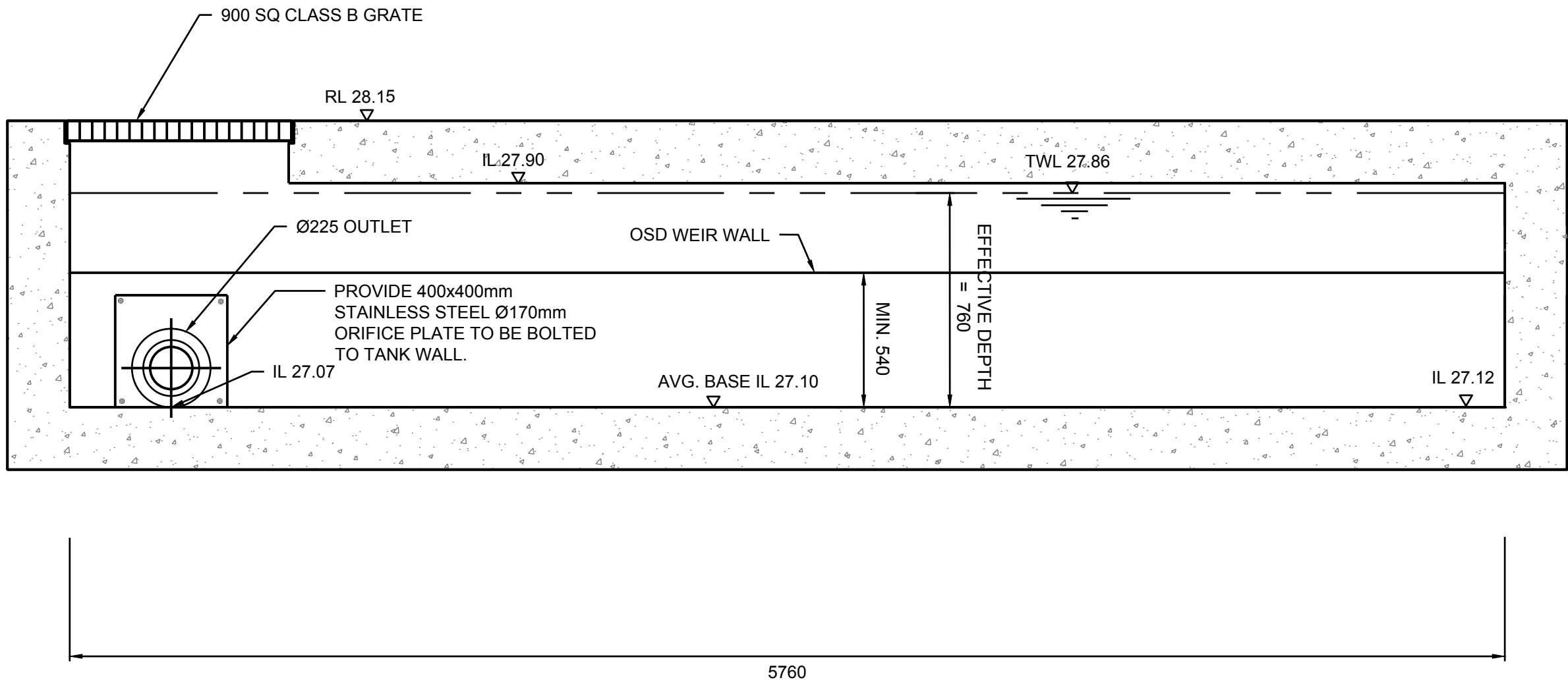
SECTION B SCALE: 1:20
