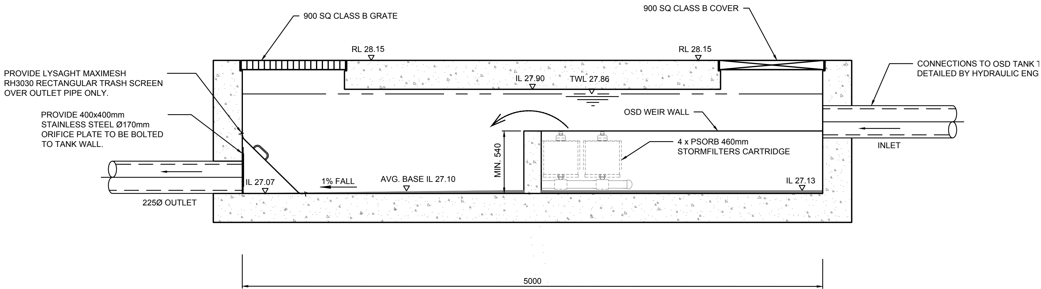
SECTION A SCALE: 1:20
