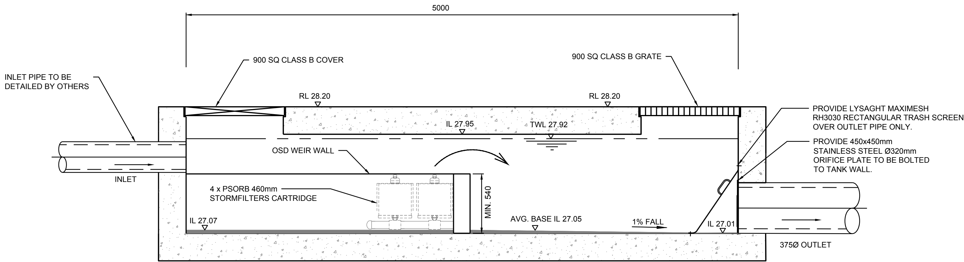
SECTION B SCALE: 1:20
