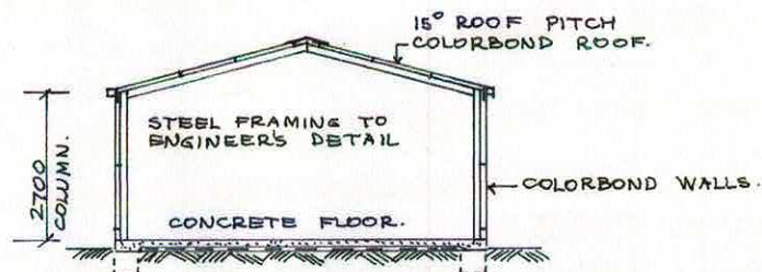
SECTION A-A 1:100
